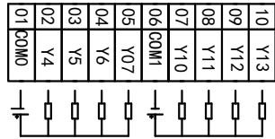
4.3寸一体机MC_20MR_6MT_i430A_FX_A接线图
